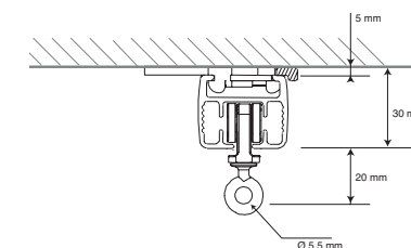
Rail cintré (sur-mesure) Jusqu'à 10 mètres (rayon de cintrage minimal de 300 cm)
